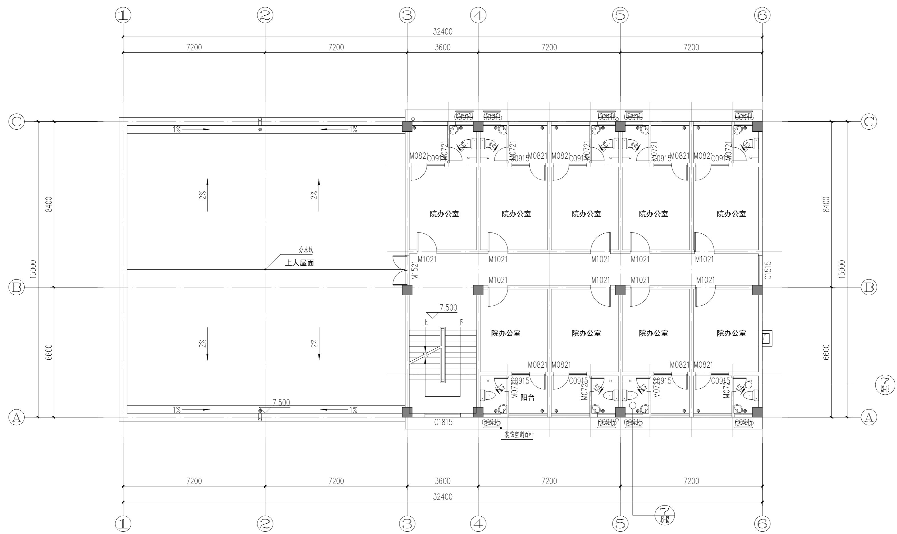
三层平面图 1:100 本层建筑面积251.97m 2
