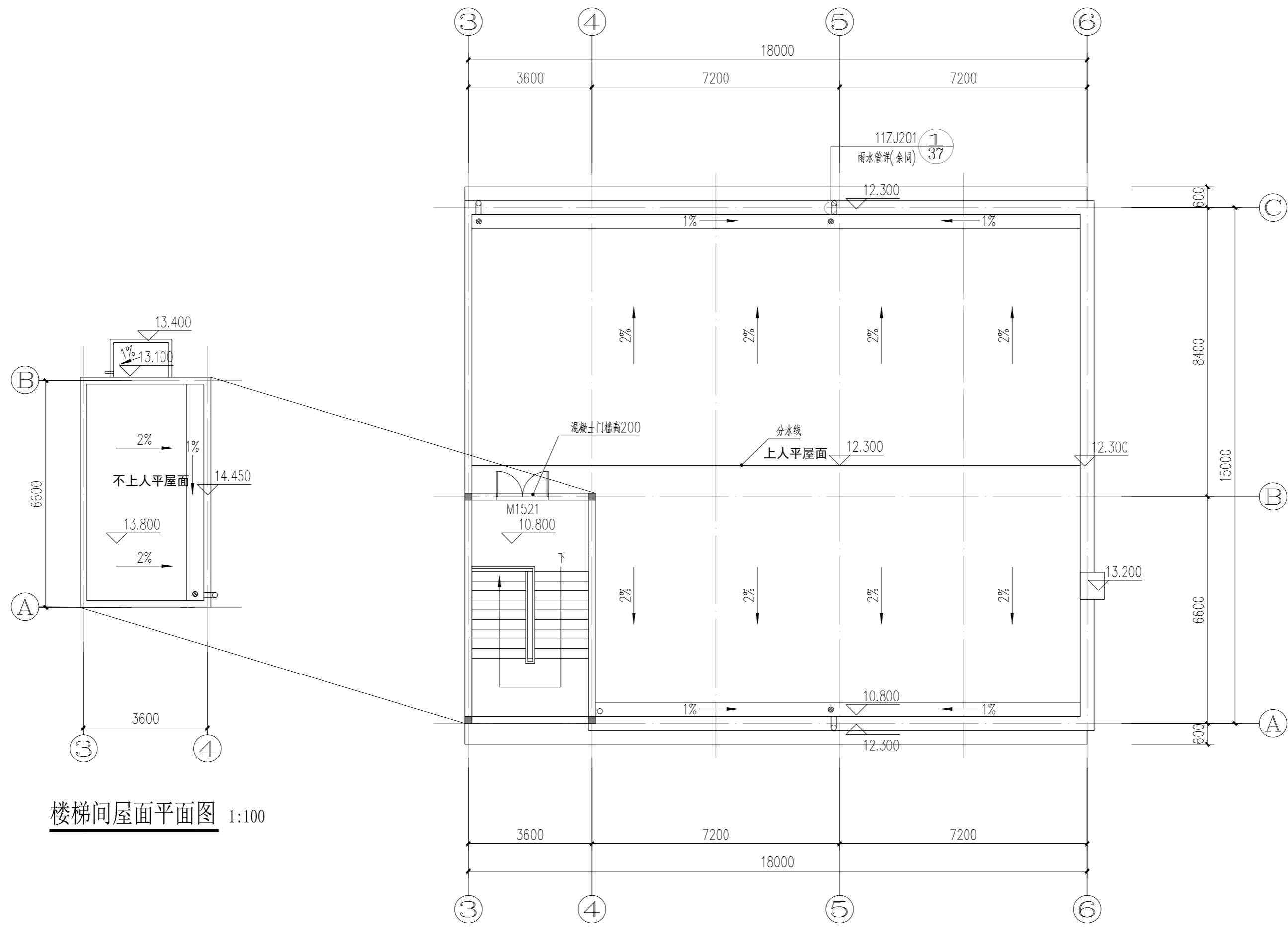
屋面平面图 1:100
