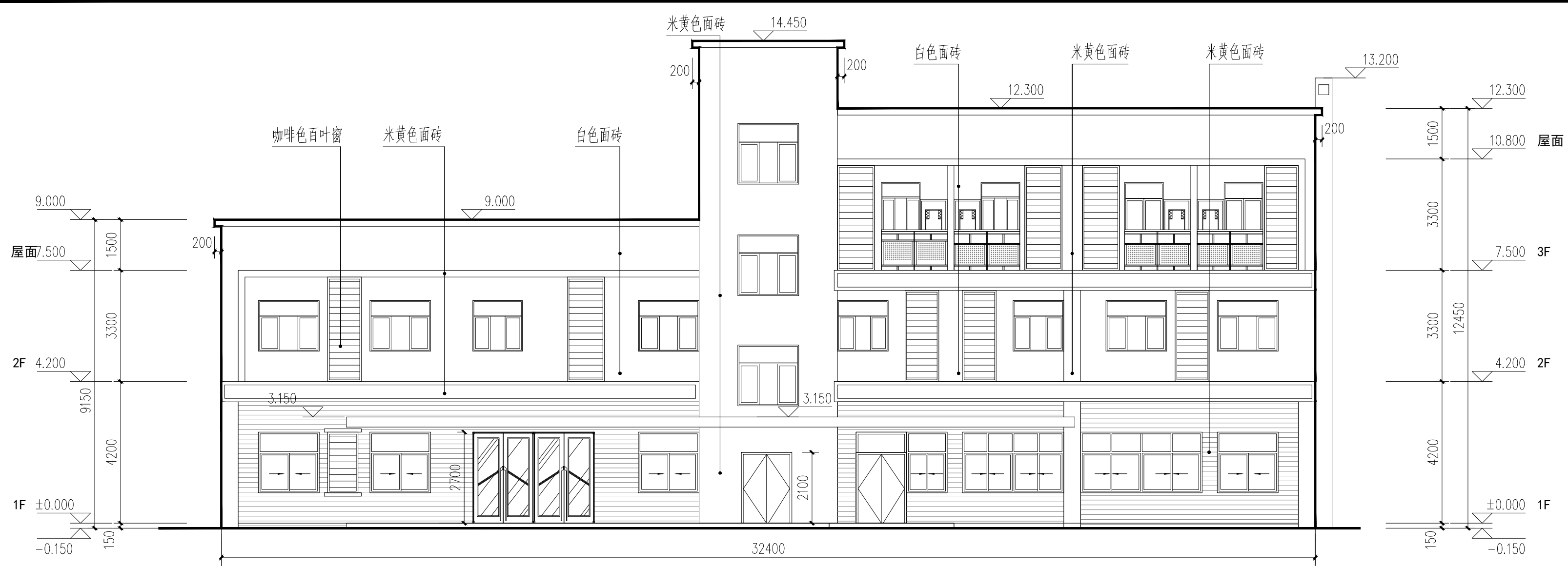
①~⑥轴立面图 1:100
