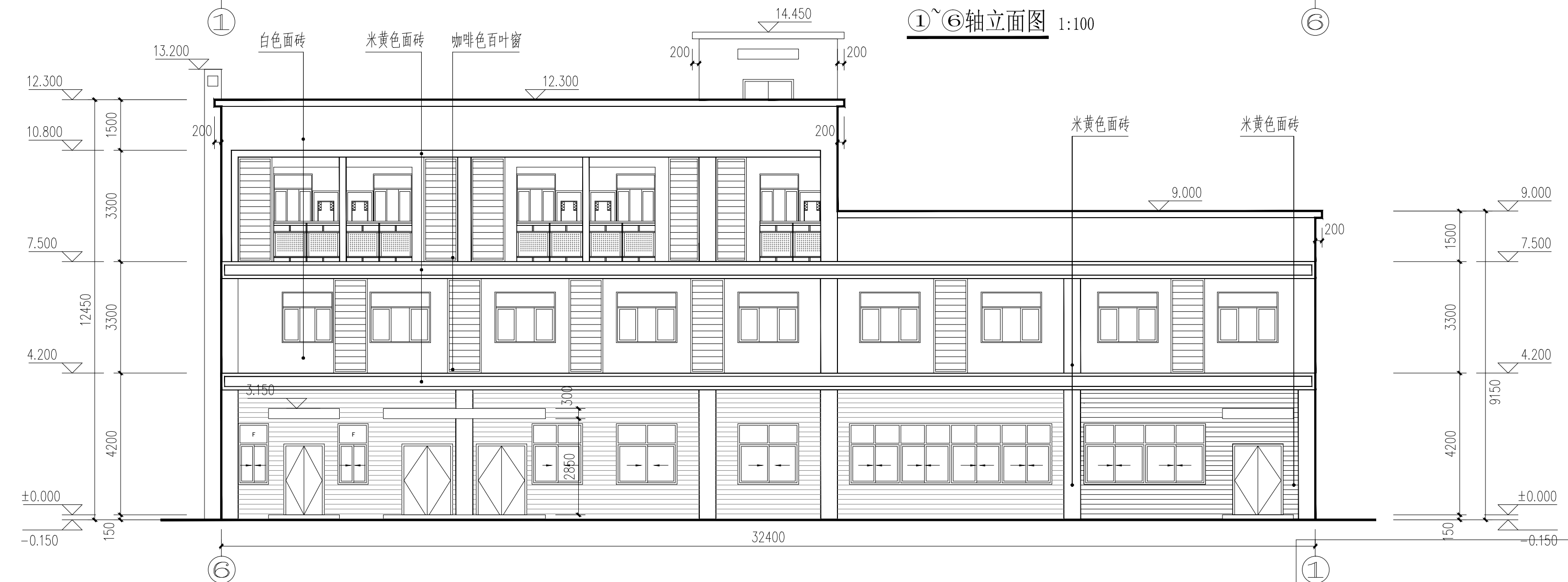
⑥~①轴立面图 1:100
