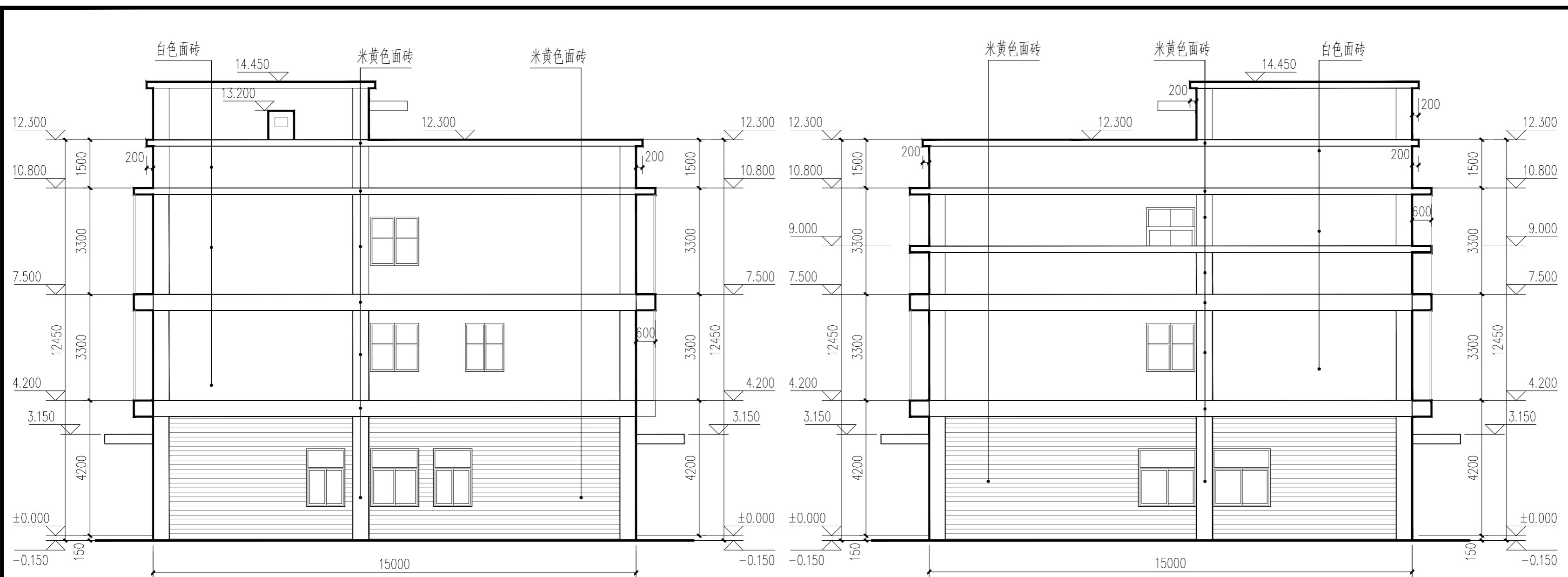
A~C轴立面图 1:100
